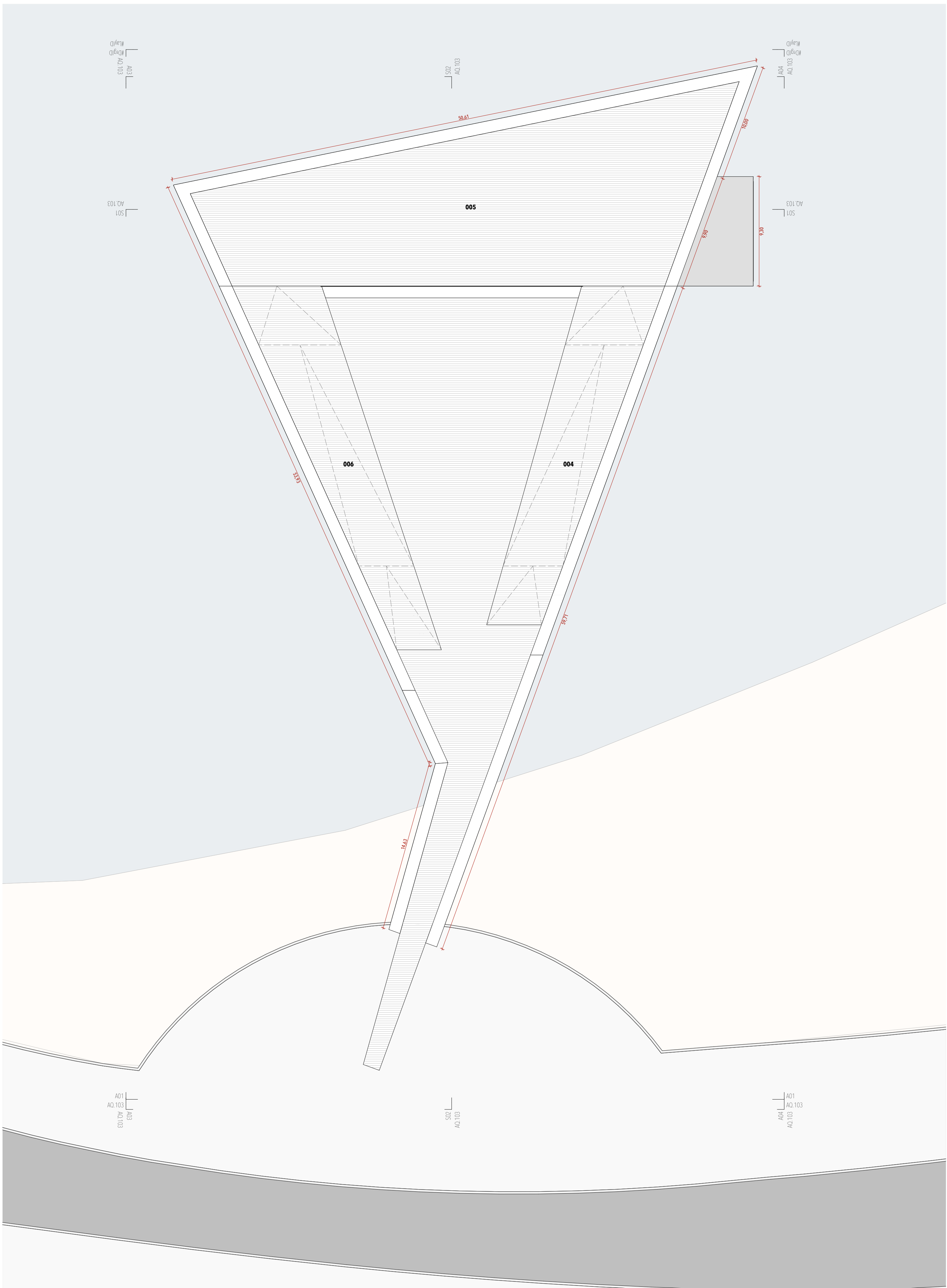
N02 NÍVEL 02 / COBERTURA 1:200
